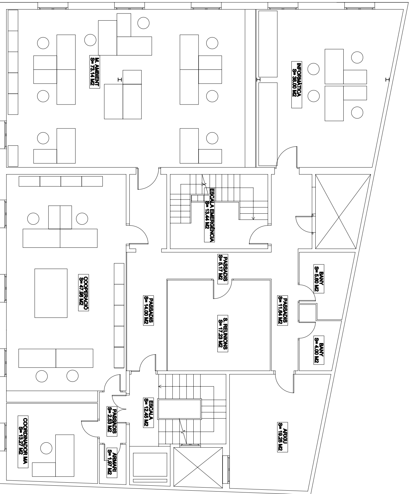
PLANTA PRIMERA E. 1/100
