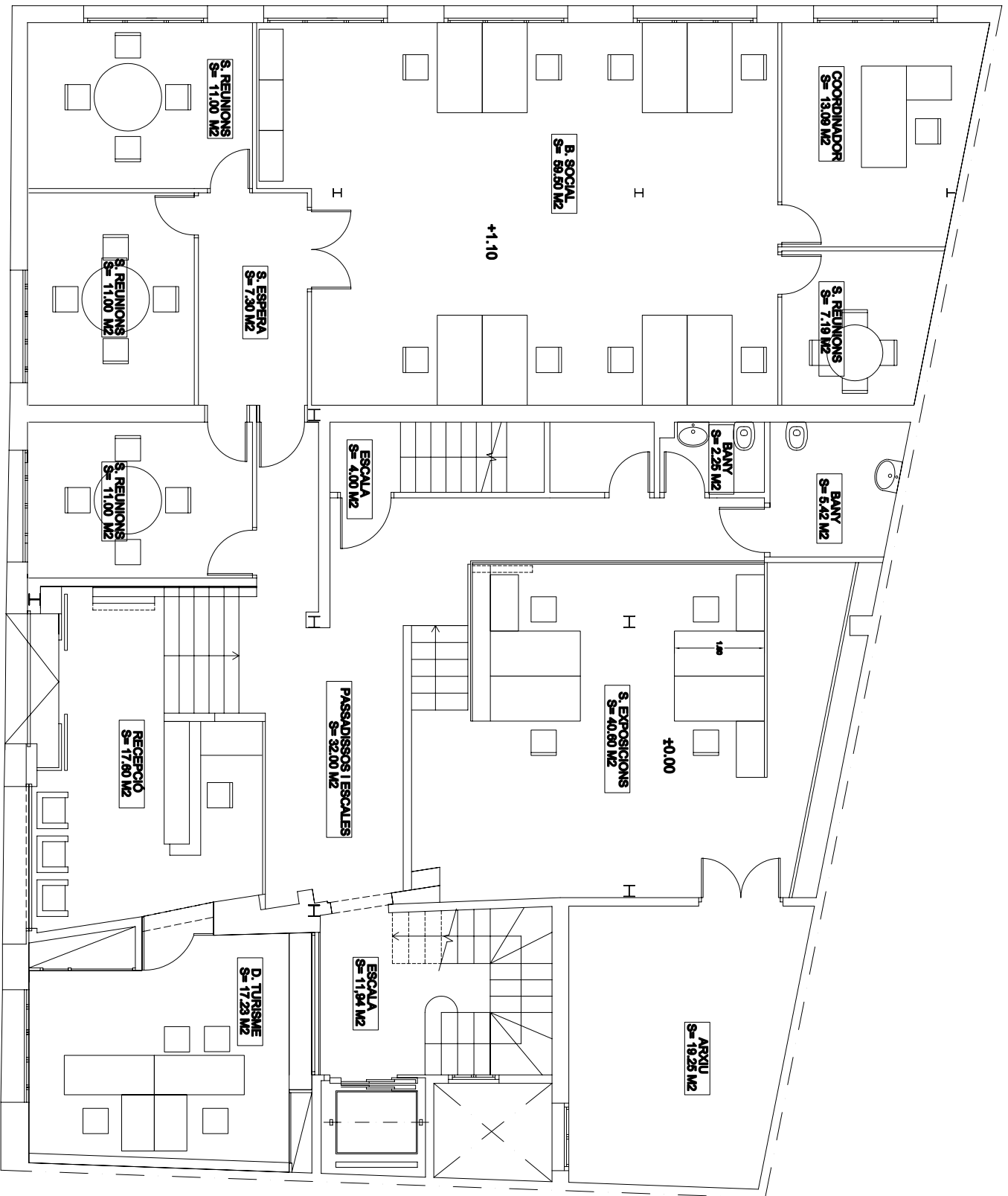
PLANTA BAIXA E. 1/100
